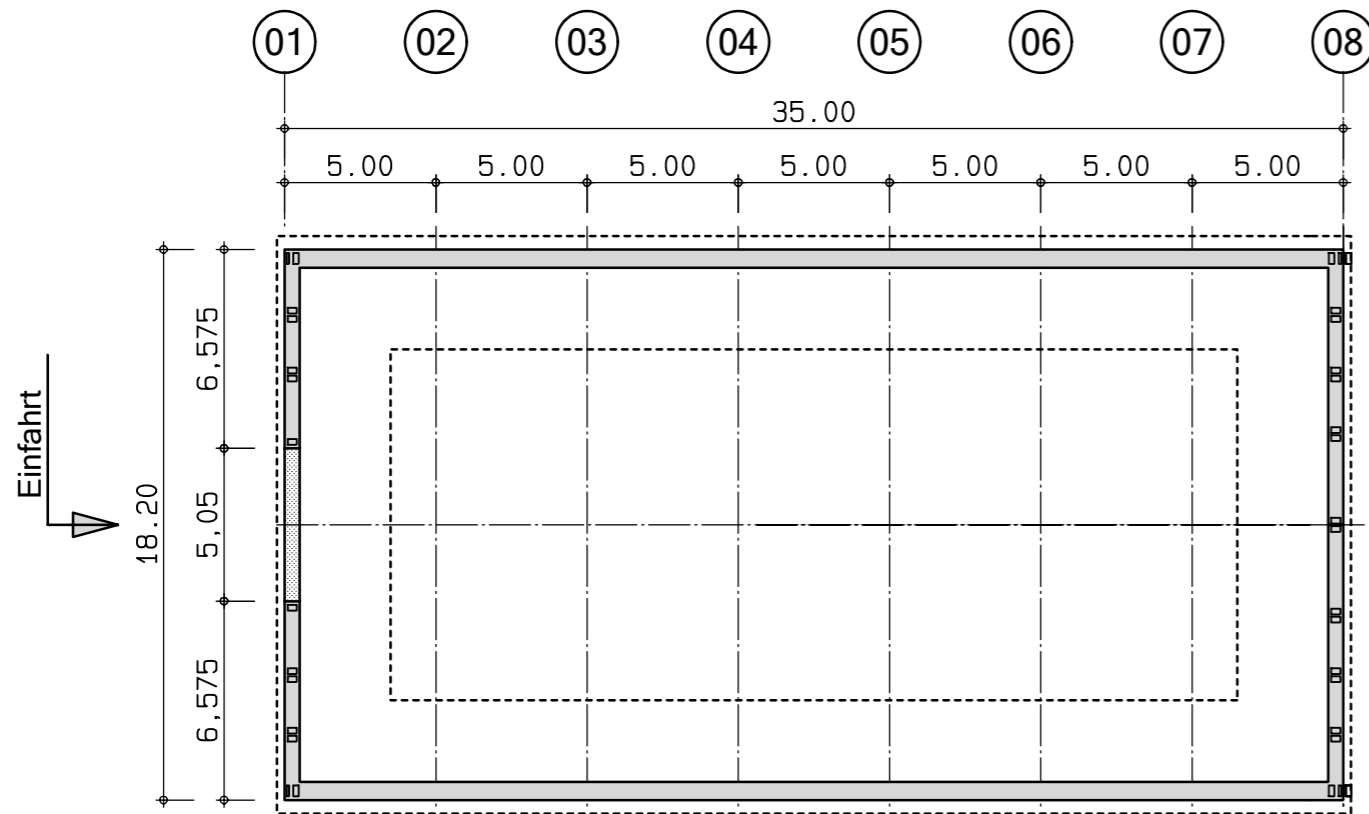
Grundriss Hallenfundament, M1:250
