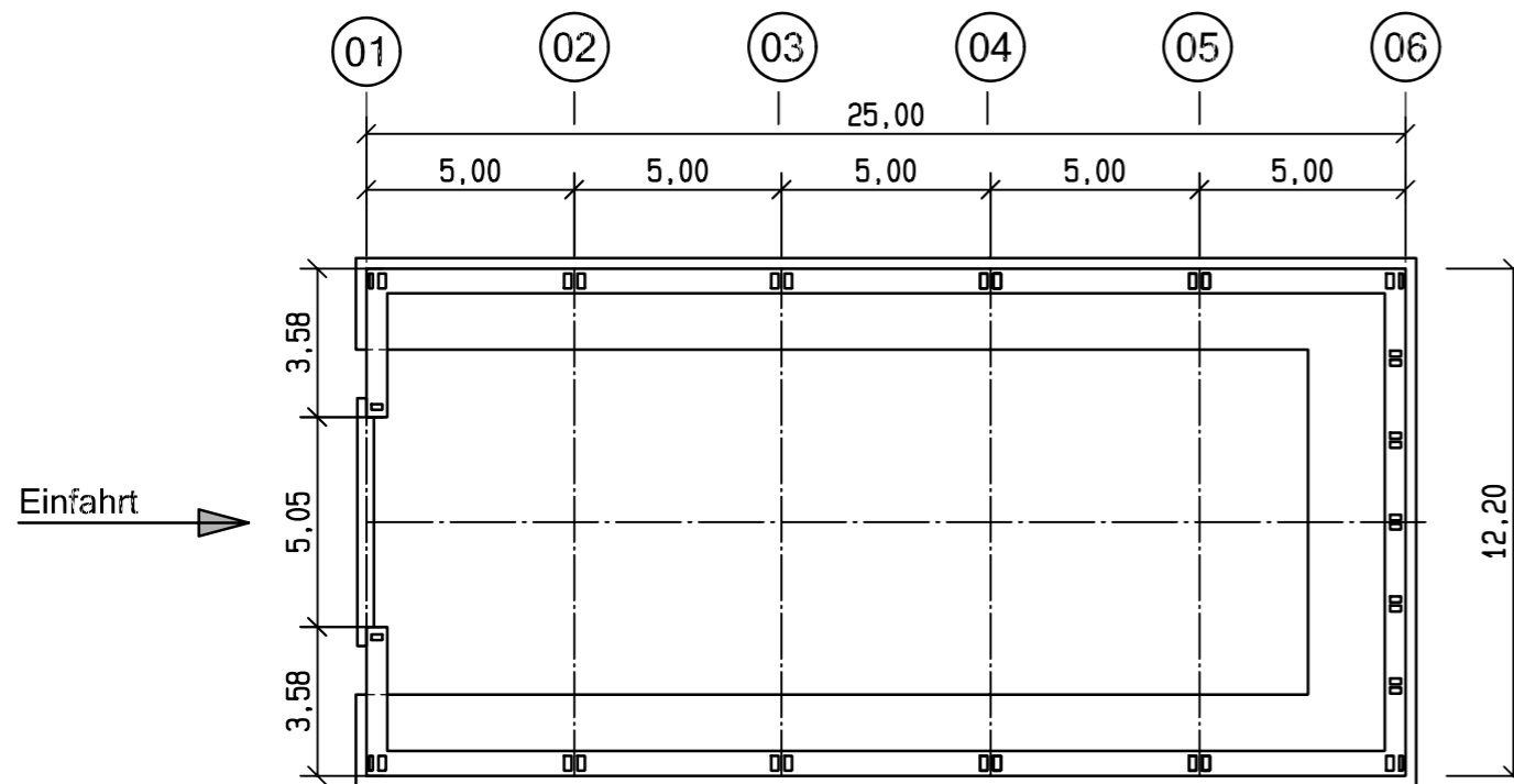
Grundriss Hallenfundament
