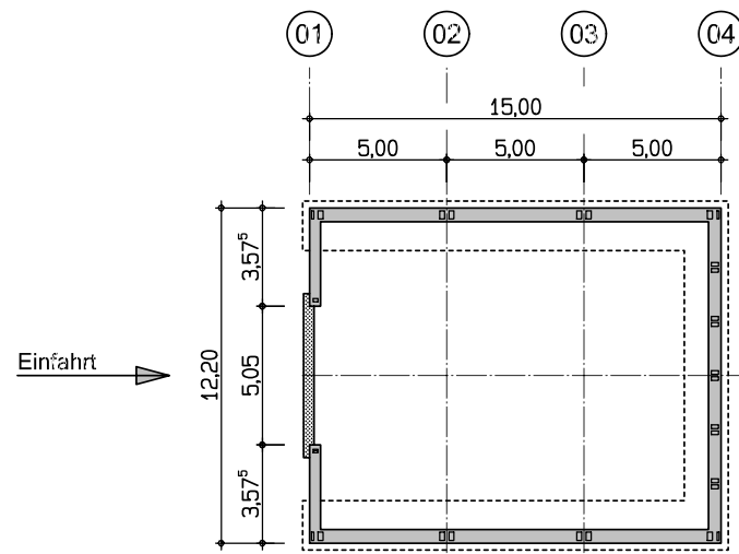
Grundriss Hallenfundament
