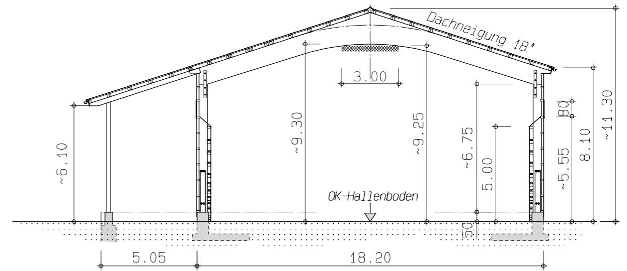
Hallenschnitt, M 1:200
