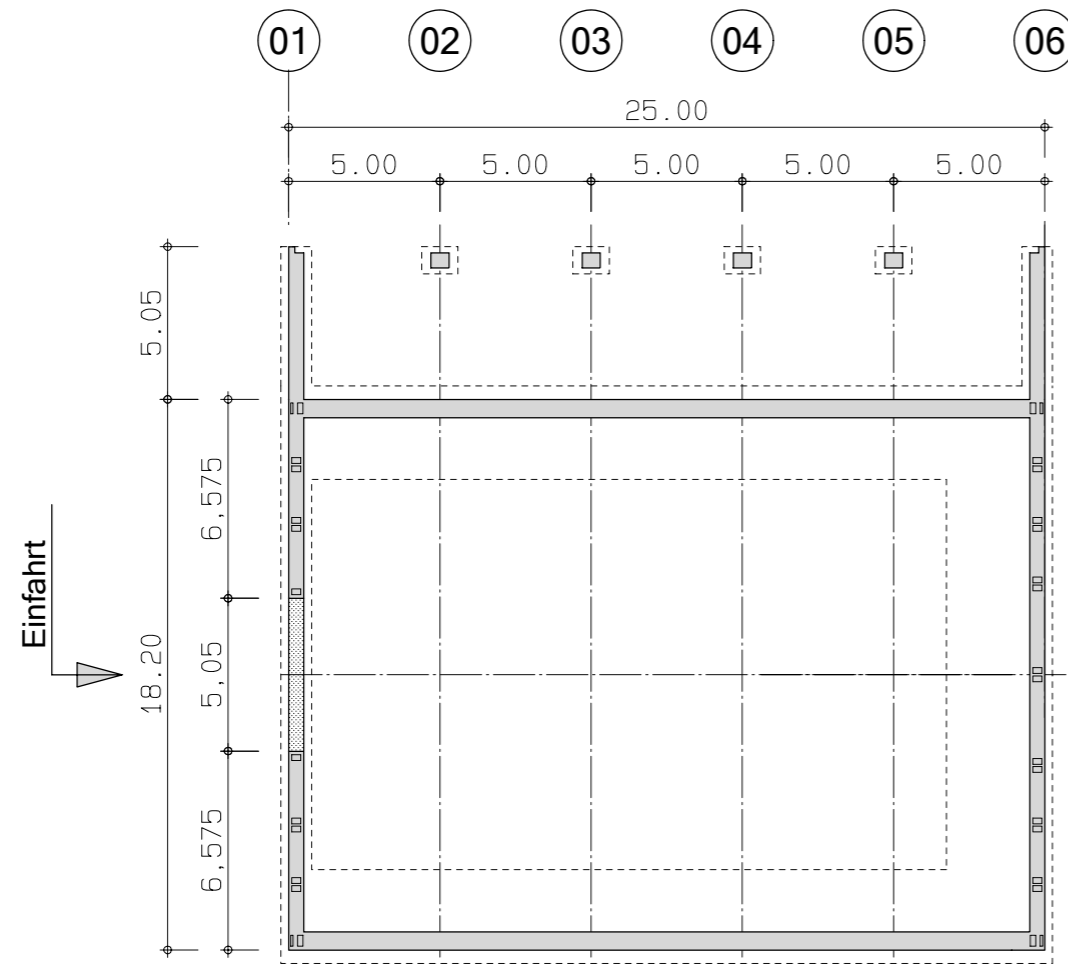
Grundriss Hallenfundament, M1:250
