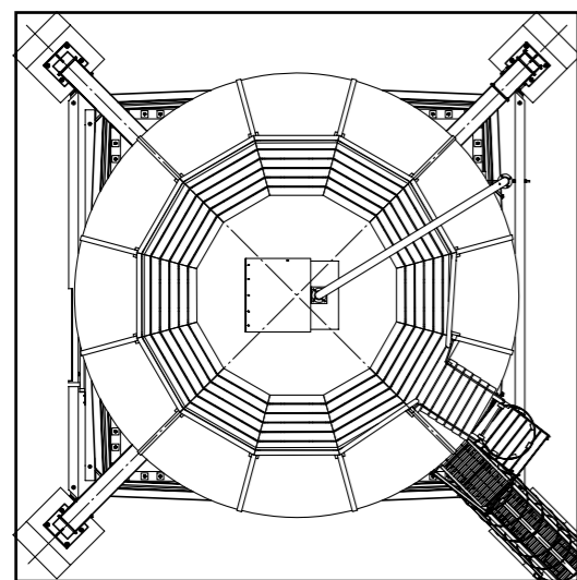
Aufstellfläche footprint
