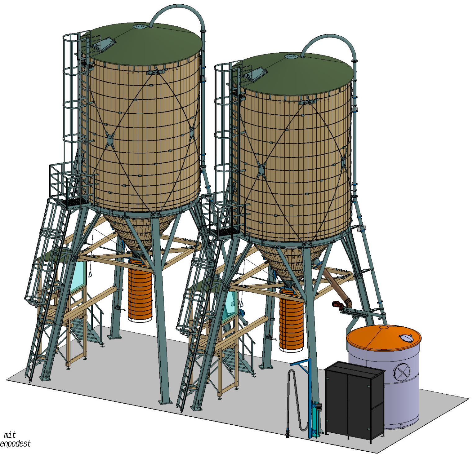
2 Streugutsilos 75 m 3 ø4.00m mit Stahlunterbau Typ N 75 400 mit Bedienungspodest Durchfahrt nebeneinander
